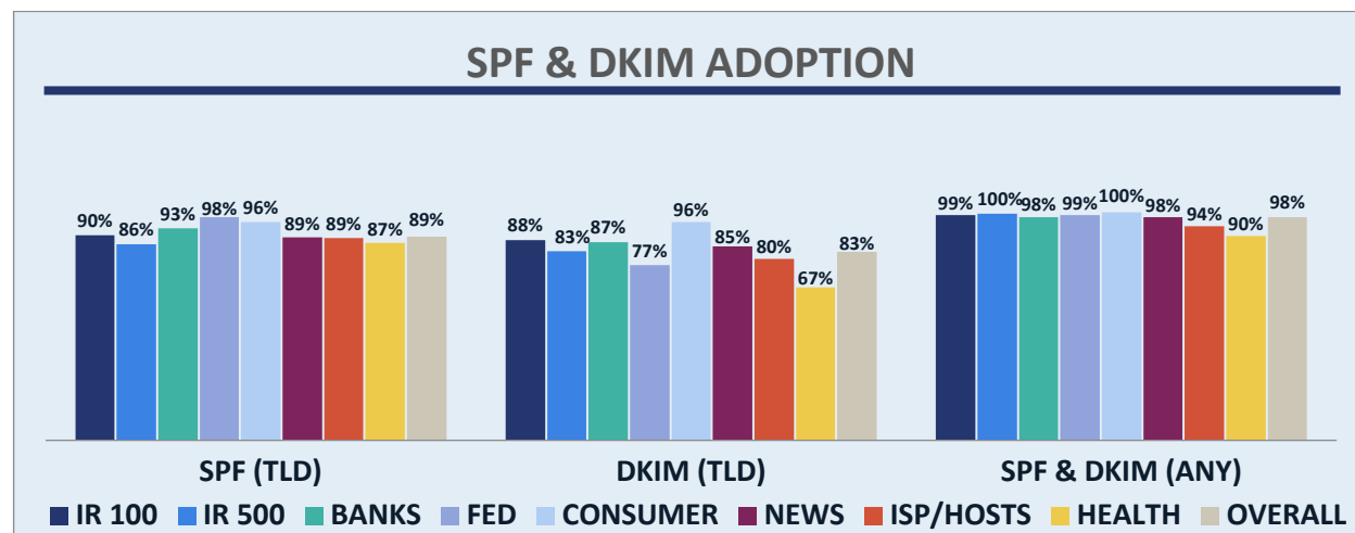
Gráfico 8. Autenticación de correo electrónico y adopción de DMARC por sector.
