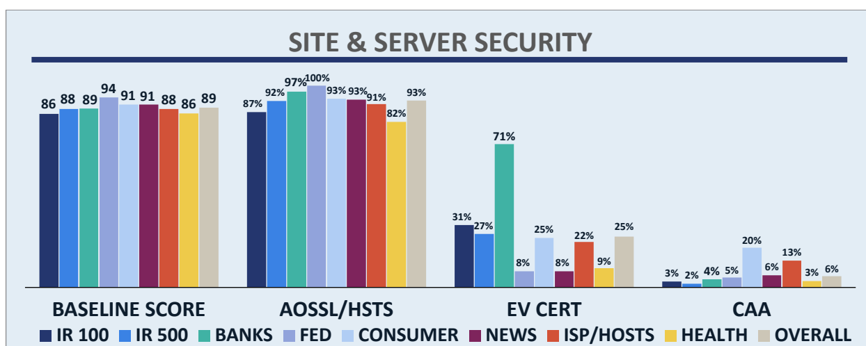
Gráfico 12. Puntuación/adopción de seguridad de sitio y servidor por sector.
